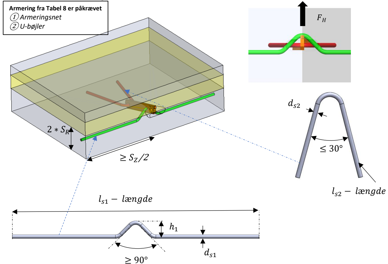
Figur 10 Armeringskrav til vipning og drejning af elementet.
