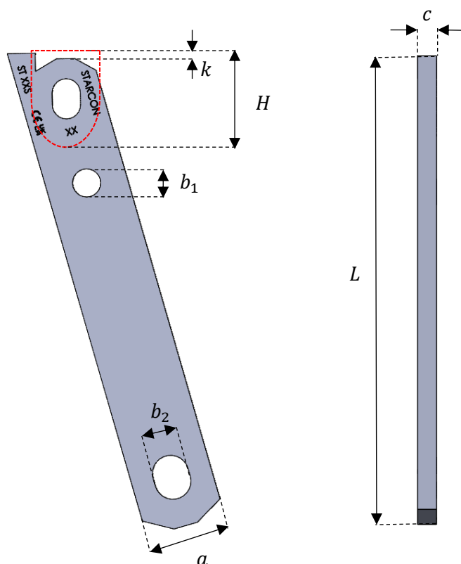
Figur 12 STA ST skitse.
