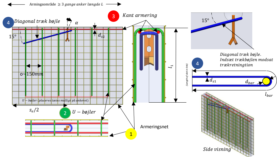
Figur 8 Armering i betonevæggen.
