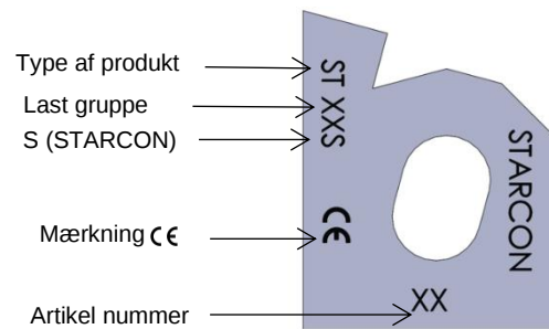
Figur 2 Mærkning på toppen af STA ST
