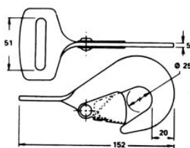
Palkrog type DPA5 Latch hook type DPA5
