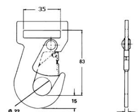
Palkrog type P50 Latch hook type P50
