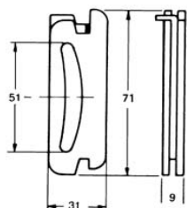
Skinnebeslag type S50 Rail buckle type S50
